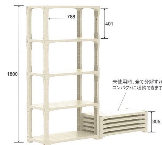
■ プラスチック棚 W900×D450×H1800 18.5kg 耐荷重:70kg(均等荷重)
